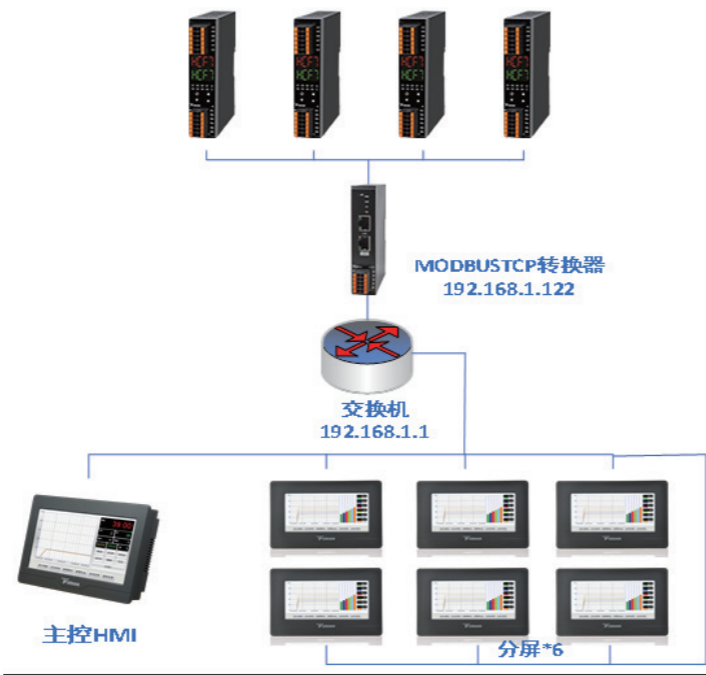
图 3 通信部分框图
