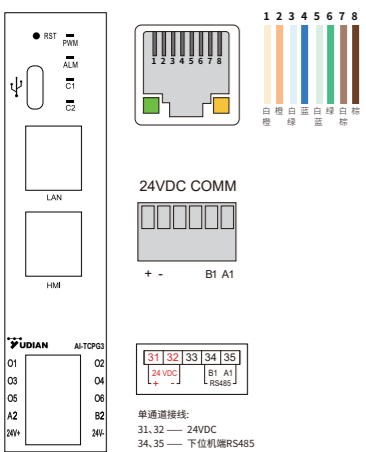
图 2 AI-Modbus-TCP 多功能通讯控制器接线图
